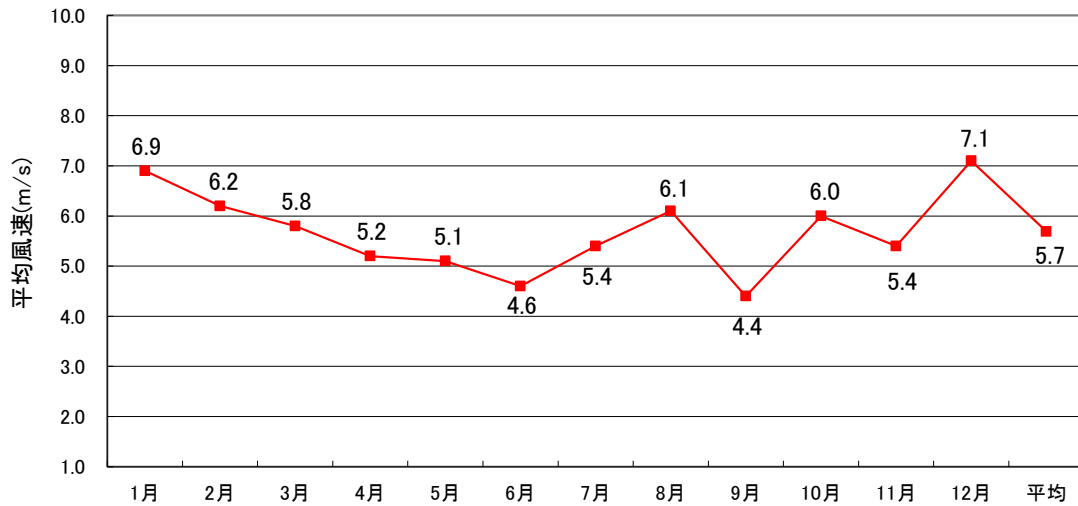
図9 月別および年間の平均風速(m/s), 風車9号機, 実測データ(地上高60m), 2014年度
