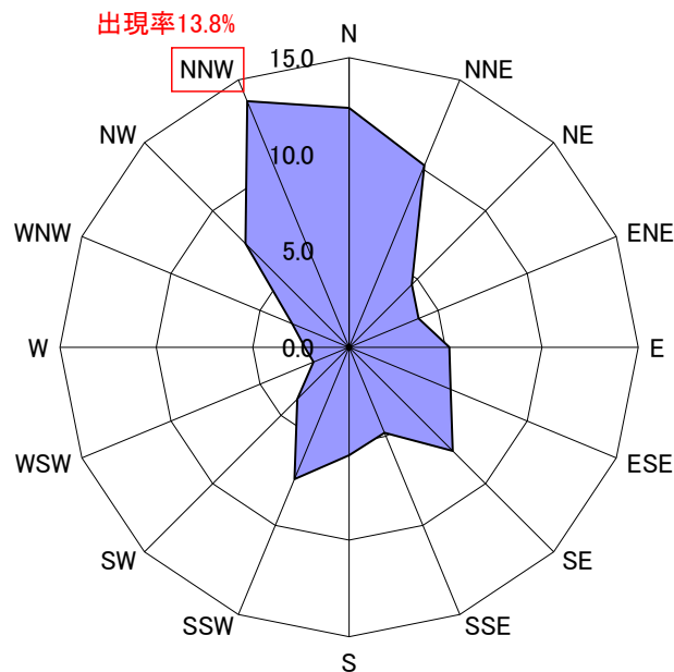
図10 年間の出現率(%), 風車9号機, 実測データ(地上高60m), 2014年度
