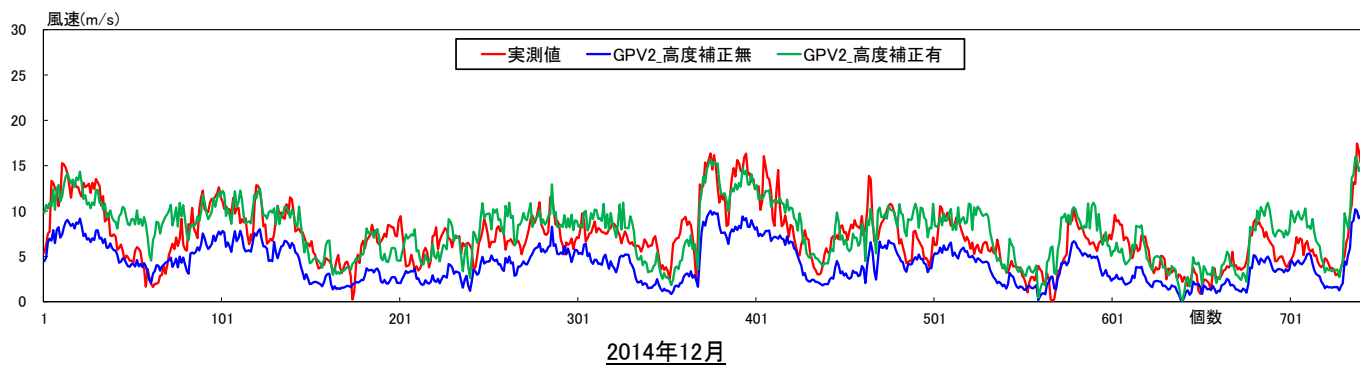
図12(続き) 実測データと気象GPVデータ(LFM-S, 地上高10m)の時系列データの比較, 図7に示すGPV2位置で取得したデータ, 風車9号機, 2014年度
