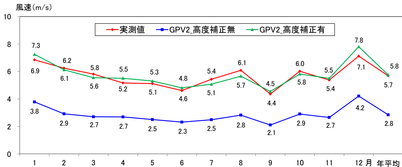
図13 実測データと気象GPVデータ(LFM-S, 地上高10m)の月別および年間における平均風速(m/s)の比較, 図7に示すGPV2位置で取得したデータ, 風車9号機, 2014年度
