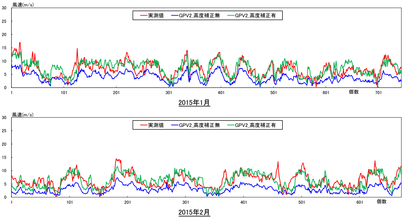
図12 実測データと気象GPVデータ(LFM-S, 地上高10m)の時系列データの比較, 図7に示すGPV2位置で取得したデータ, 風車9号機, 2014年度
