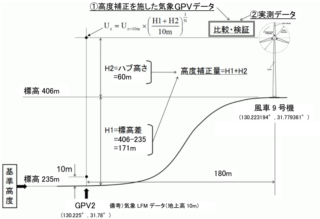
図11 気象GPVデータ(LFM-S, 地上高10m)に基づいた簡易風況推定法の概念図
