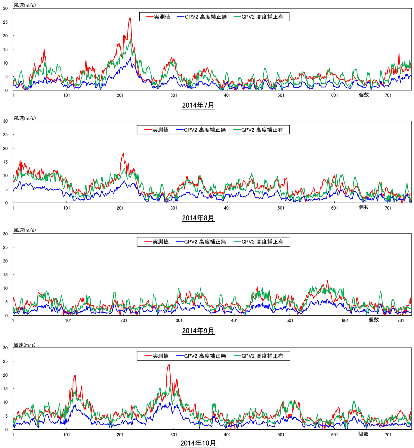
図12(続き) 実測データと気象GPVデータ(LFM-S, 地上高10m)の時系列データの比較, 図7に示すGPV2位置で取得したデータ, 風車9号機, 2014年度
