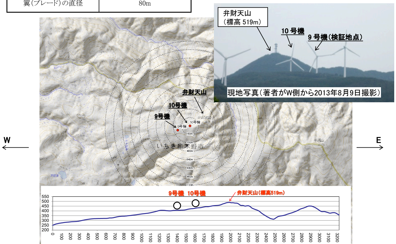
図4 串木野れいめい風力発電所9号機(含10号機)周辺地形(数値データ)、東西方向の地形断面と現地写真
