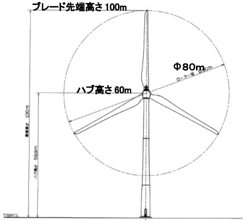
図5 風車の仕様
